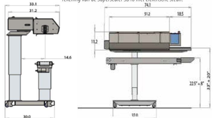
Tekening van de Supersealer SB40 met elektrische steun.
